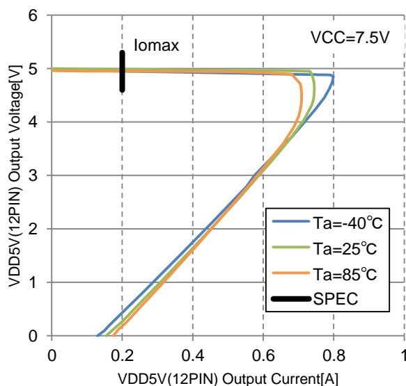
Fig10. [VDD] Vo vs. Io@VCC=7.5V
