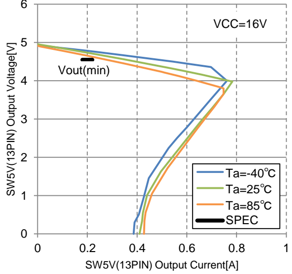
Fig46. [SW5V] Vo vs. Io@VCC=16V
