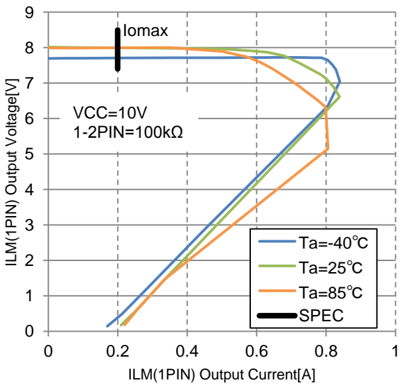
Fig26. [ILM(8V)] Vo vs. Io@VCC=10V
