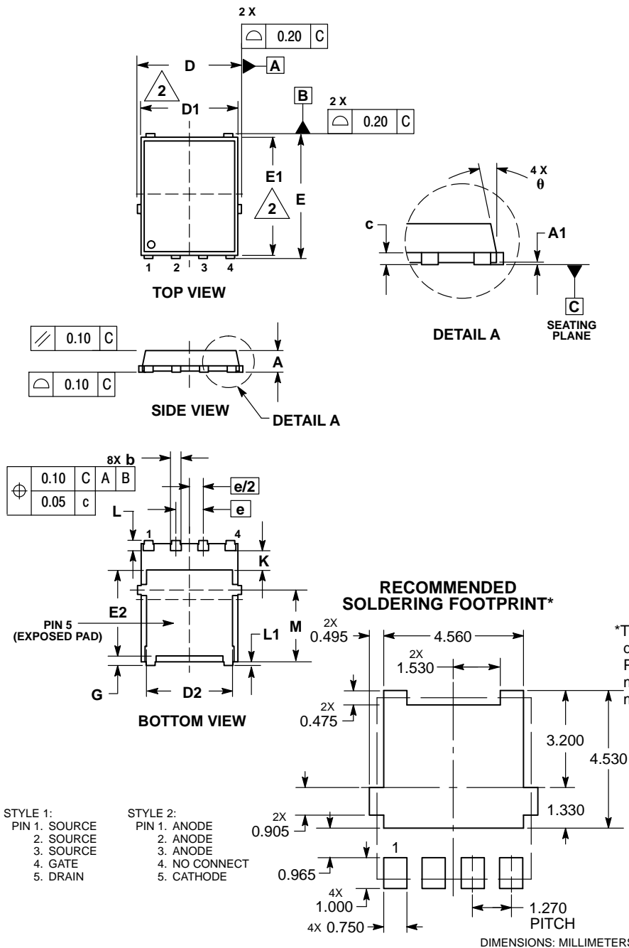
1 SCALE 2:1
