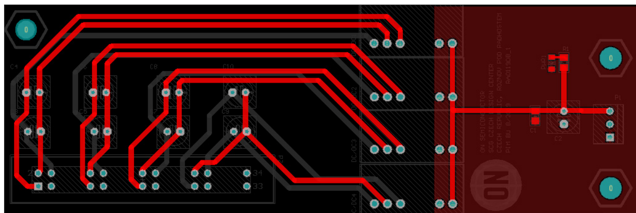
Figure 20. Top Layer
