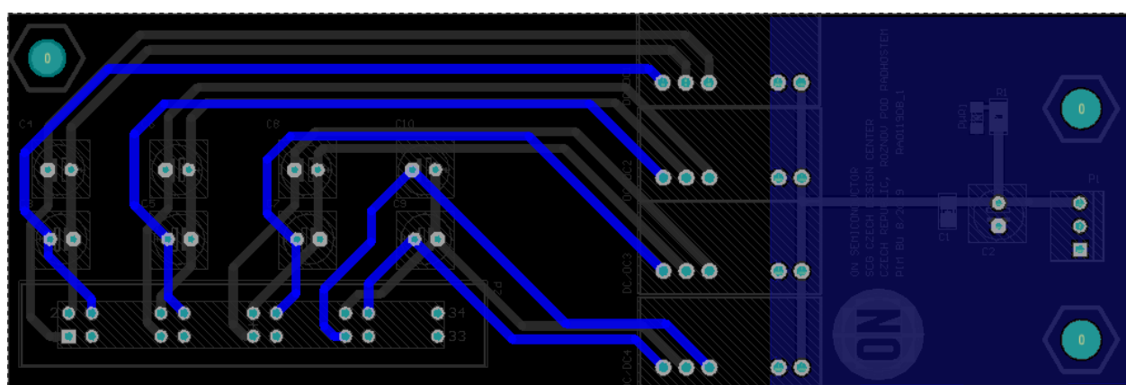
Figure 21. Bottom Layer
