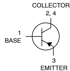
SOT-223 CASE 318E STYLE 1
