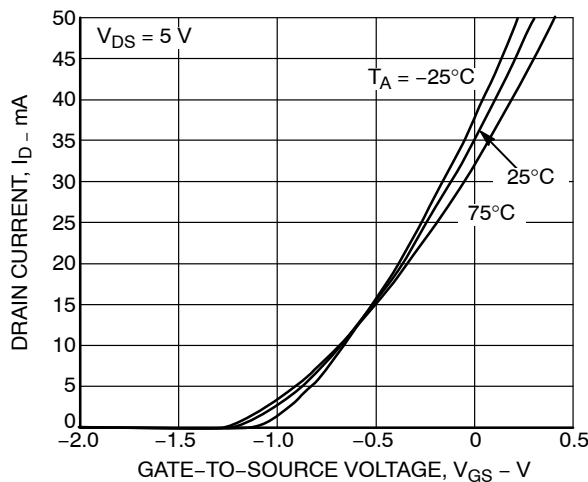
Figure 4. I_D - V_{GS}
