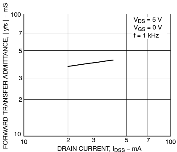
Figure 6. |y_{fs}| - I_{DSS}
