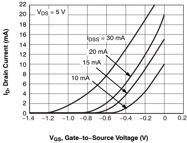
Figure 3. I_D - V_{GS}
