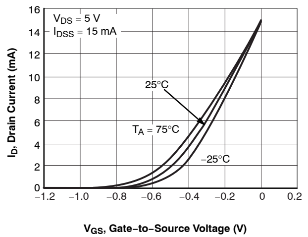
Figure 4. I_D - V_{GS}
