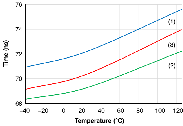
(1) t_{DIS}, V_{DD1} = 3.3V (2) t_{DIS}, V_{DD1} = 5V (3) t_{DIS}, V_{DD1} = 20V
