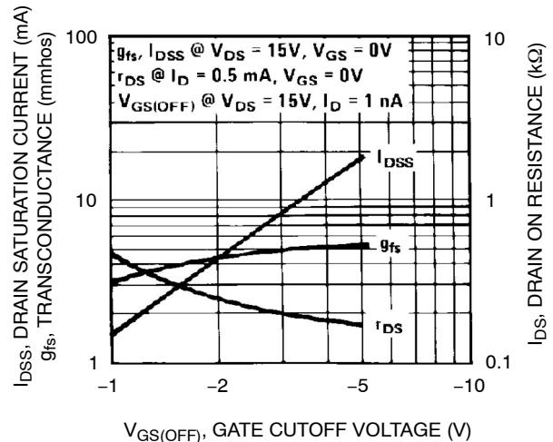
Figure 6. Parameter Interaction
