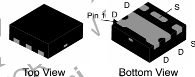
MicroFET (UDFN6) CASE 517DV
