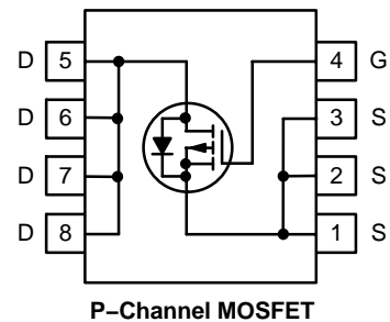
P-Channel MOSFET
