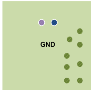
Figure 23. Layer 1
