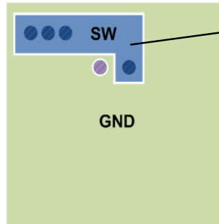
Figure 24. Layer 3
