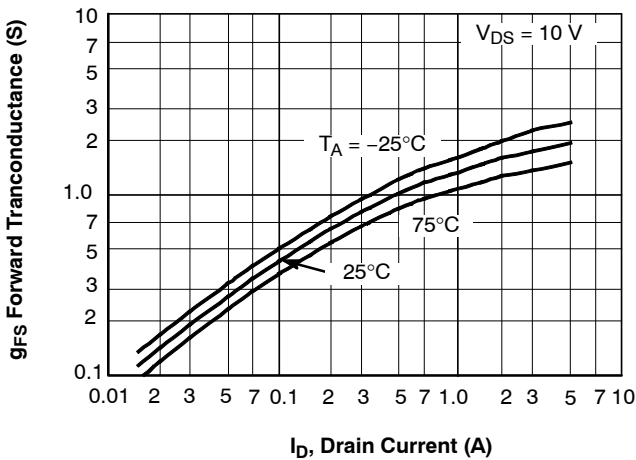
Figure 6. g_{FS} - I_D
