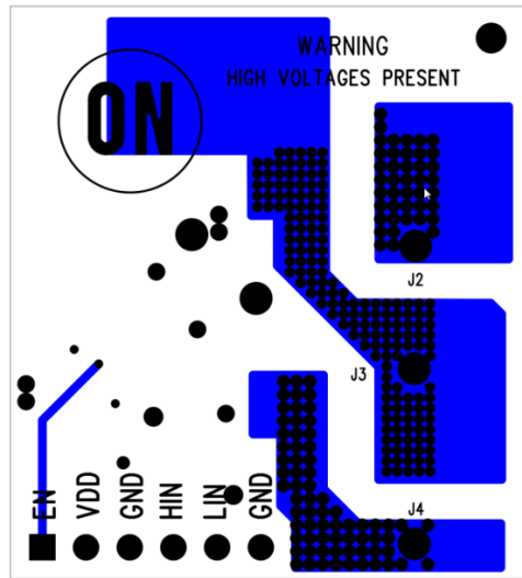
Bottom Layer
