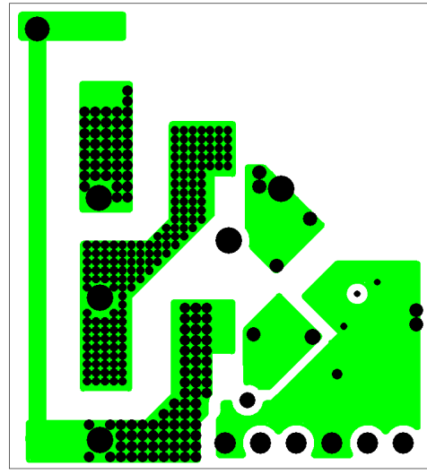
Layer 2, Internal
