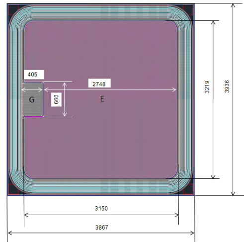
DIE OUTLINE
