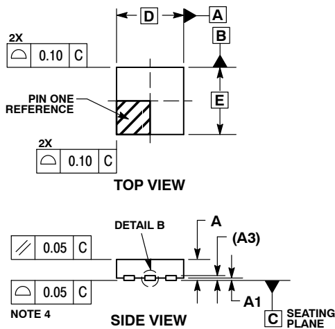
SCALE 4:1
