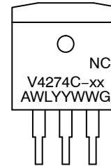
D2PAK DS SUFFIX CASE 418AF
