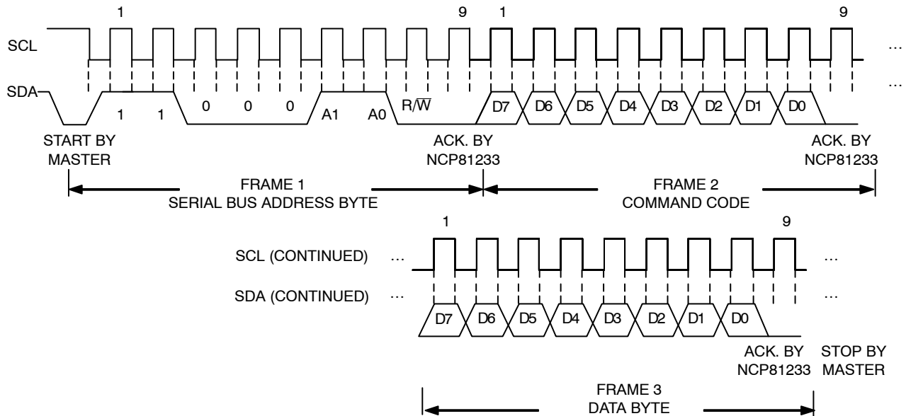
Figure 20. Write Byte
