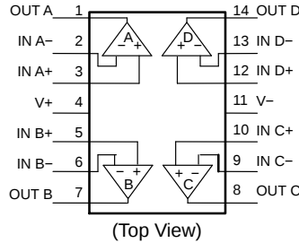
SOIC-14
