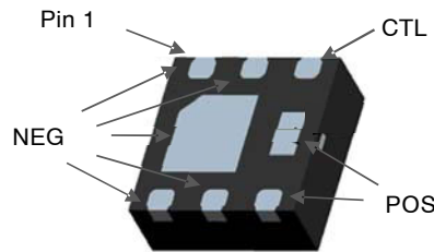
MicroFET 2x2 mm
