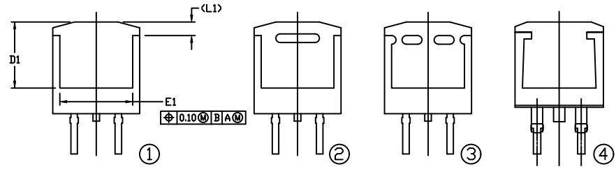
VIEW A-A
