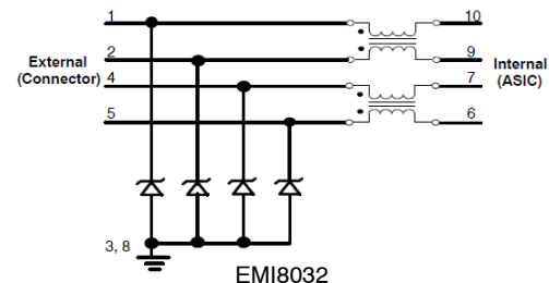
EMI8032
