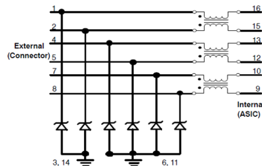
EMI8033
