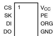
SOIC (V) and TSSOP (Y)
