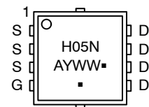
WDFN8 ( \mu 8FL) CASE 511AB
