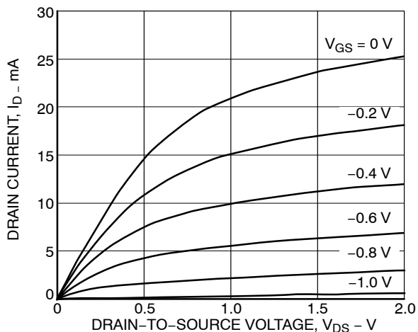
Figure 1. I_D - V_{DS}
