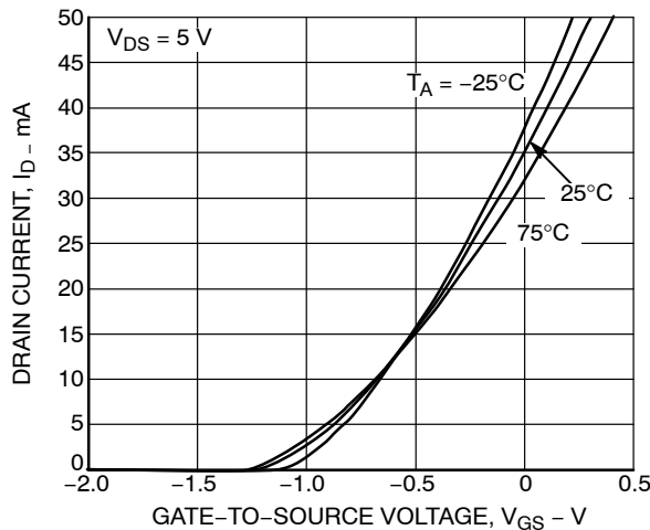
Figure 4. I_D - V_{GS}
