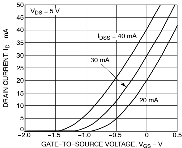
Figure 3. I_D - V_{GS}
