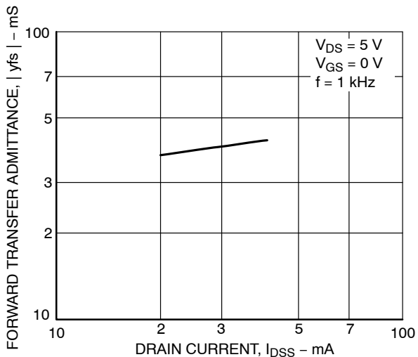
Figure 6. |y_{fs}| - I_{DSS}
