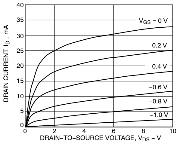
Figure 2. I_D - V_{DS}
