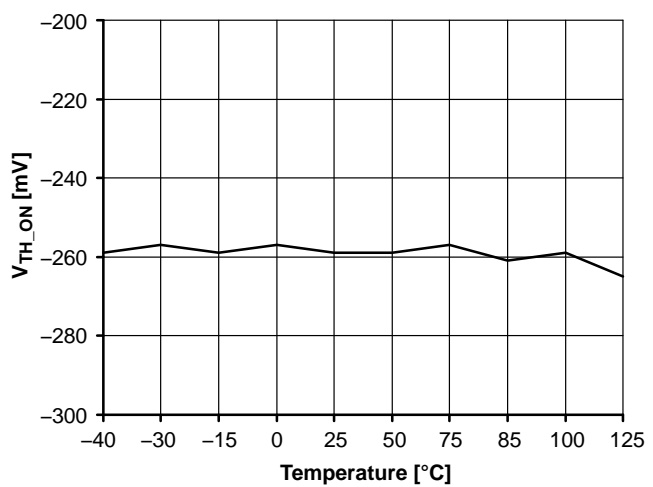
Figure 8. V TH_ON
